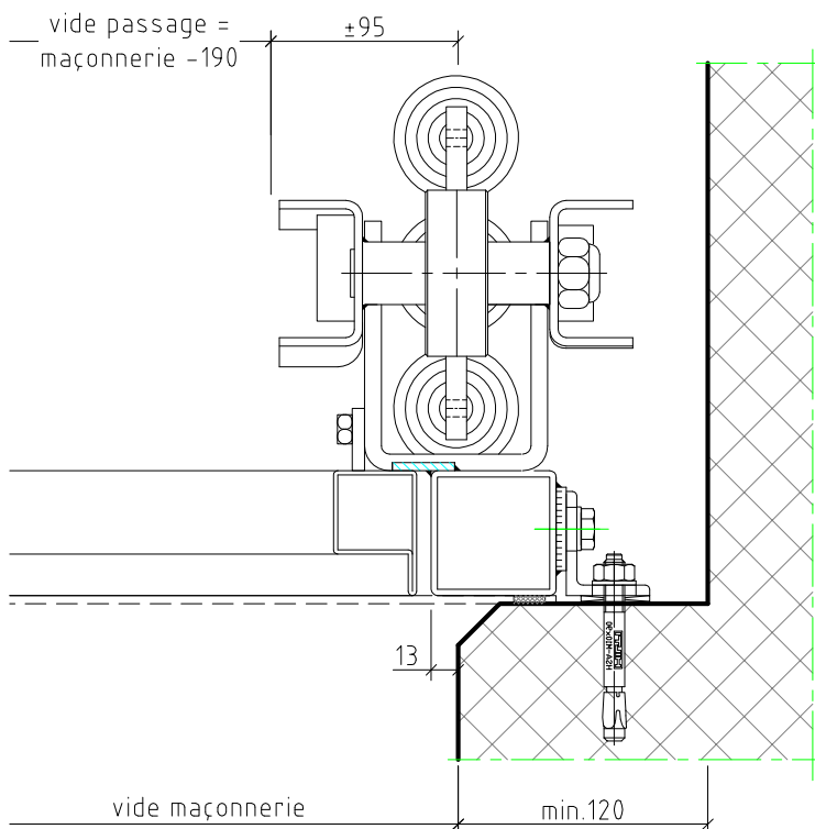
Détail D
