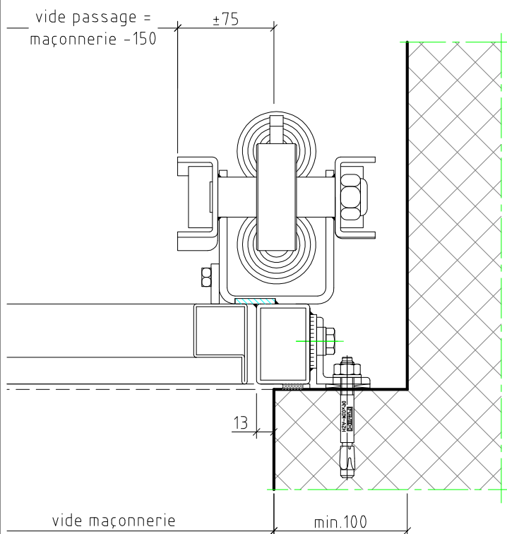
Détail C
