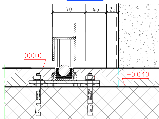
Détail F
