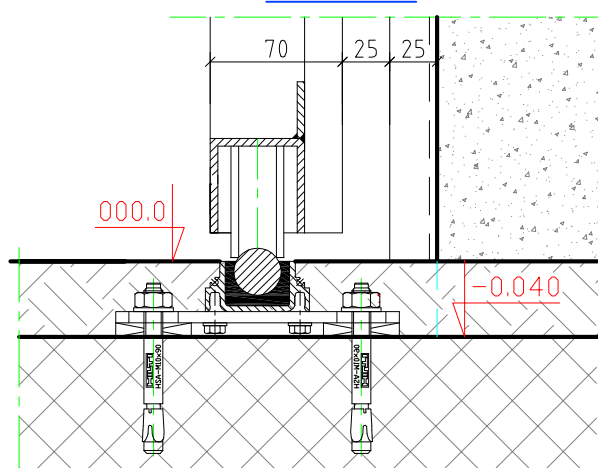
Détail D
