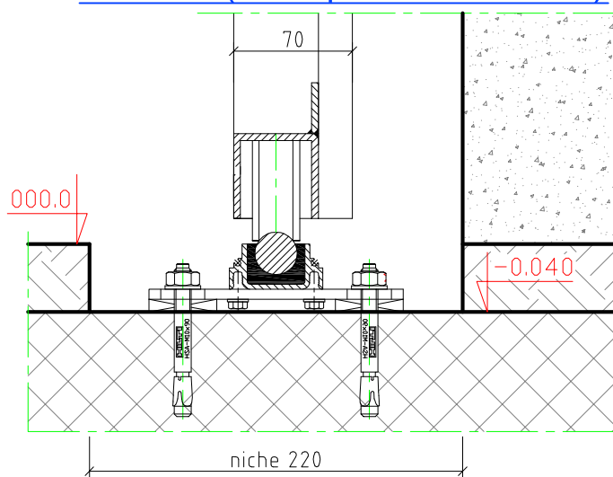
Détail A (avec porte de service)
