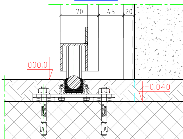
Détail E
