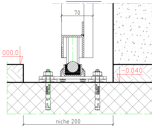
Détail B
