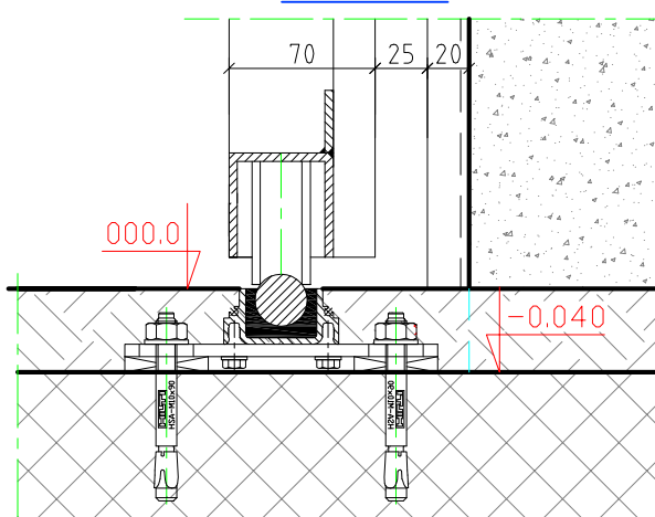
Détail C
