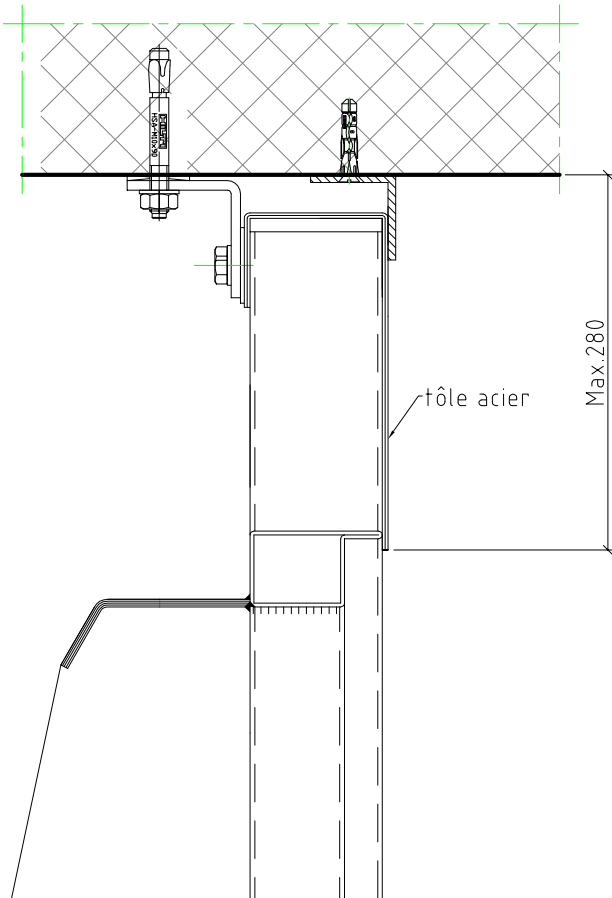
Détail A
