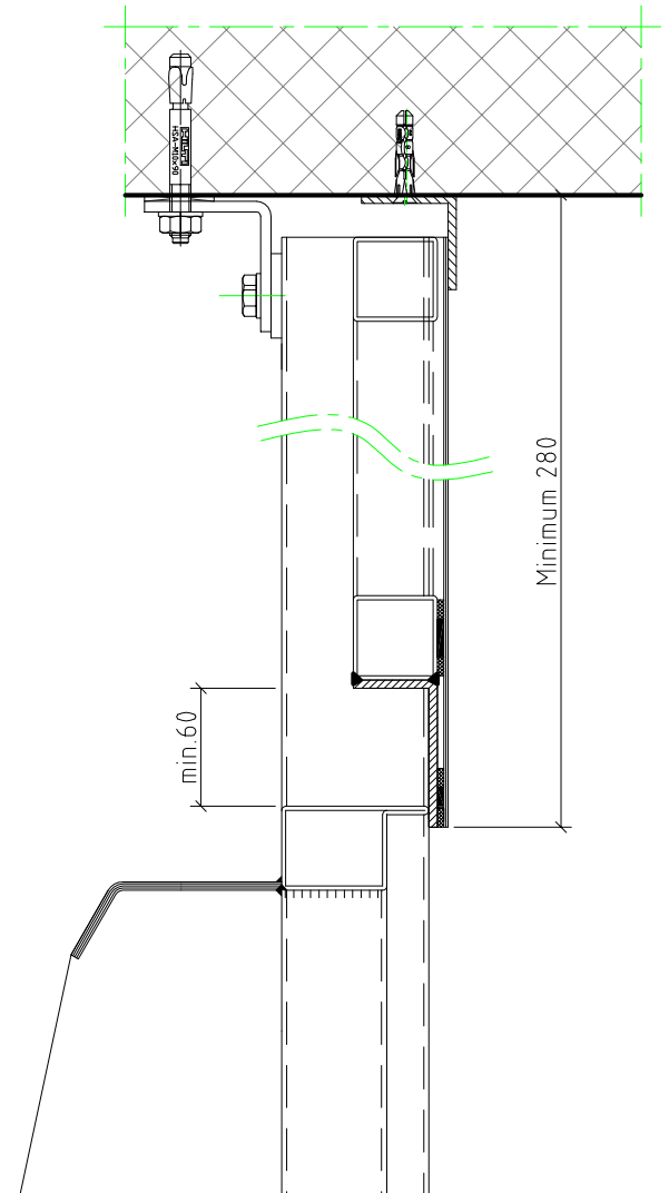
Détail B
